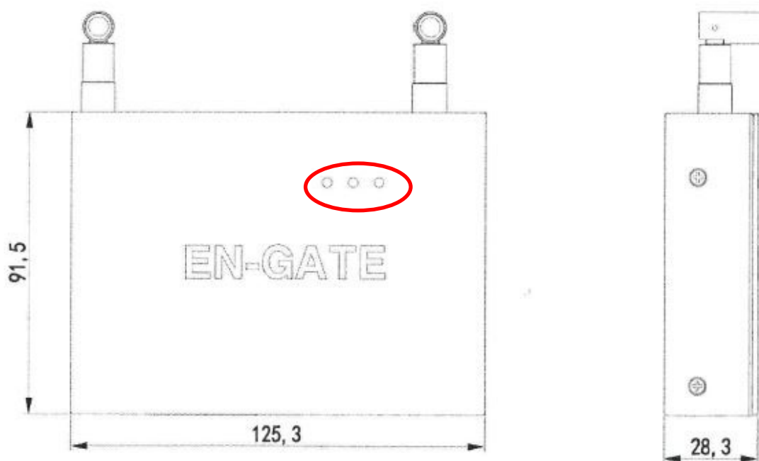
Figura 379 - Dimensioni dispositivo
