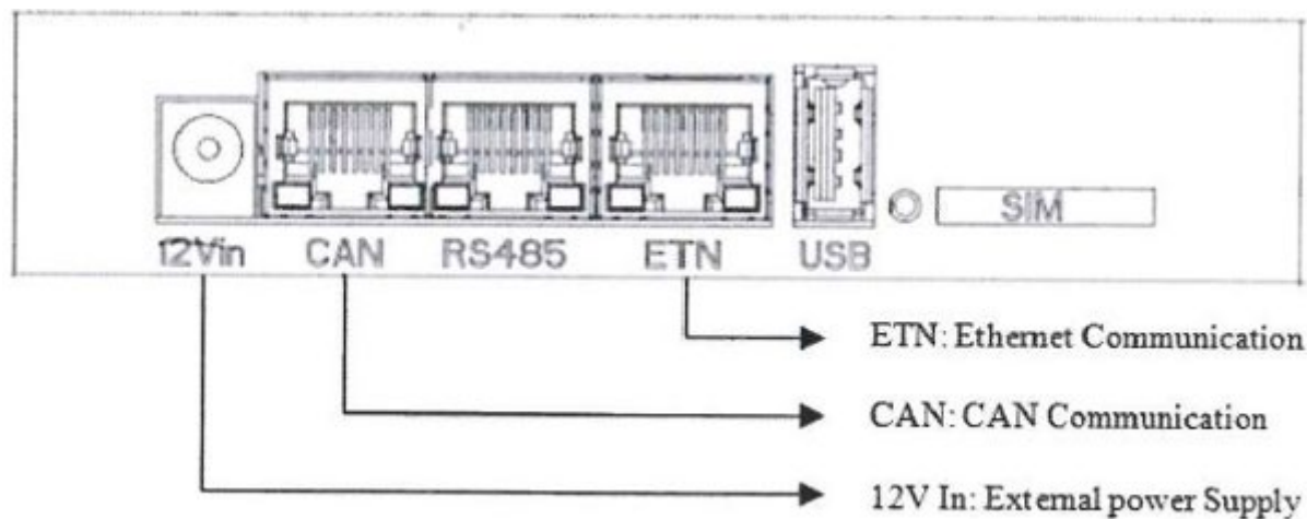
Figura 38 - Definizione ingressi
