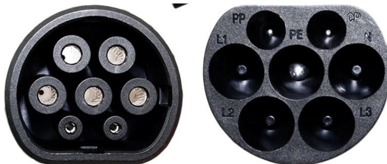
Figura 6 - Connettore Type2
