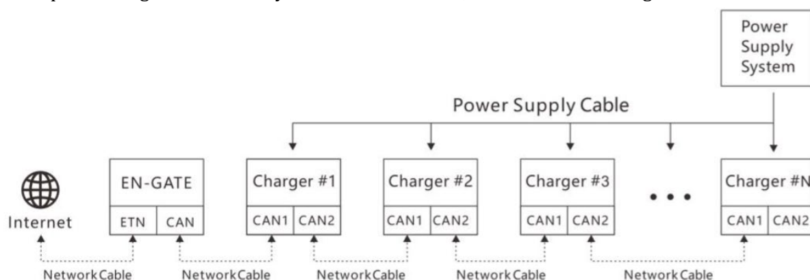
Figura 37 - Collegamento tra ZVM-GATEWAY e caricatori
